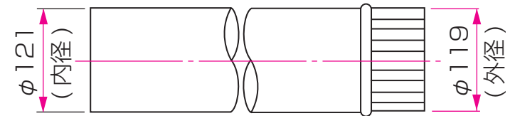
排気筒差し込み部詳細
