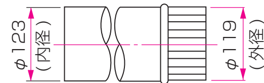
Ⓜ 排気筒アダプタ差し込み部詳細
